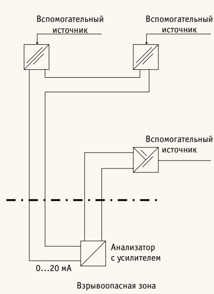
Рис. 10. Пример схемы с нелинейными элементами
